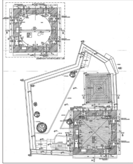
Plan 4. Çinili Sıbyan Mektebi planı (İstanbul 6 Numaralı Kültür Varlıklarını Koruma Bölge Kurulu Müdürlüğü'nden alınan 2016 tarihli rölövede bulunan plan)
