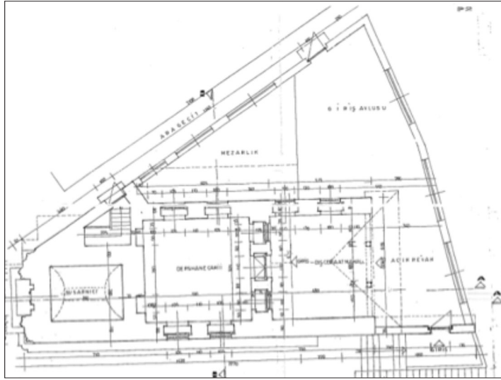
Plan 5. Kapı Ağası Yakup Ağa Sıbyan Mektebi planı. (İstanbul 6 Numaralı Kültür Varlıklarını Koruma Bölge Kurulu Müdürlüğü'nden alınan 2012 tarihli restitüsyon raporunda bulunan plan)
