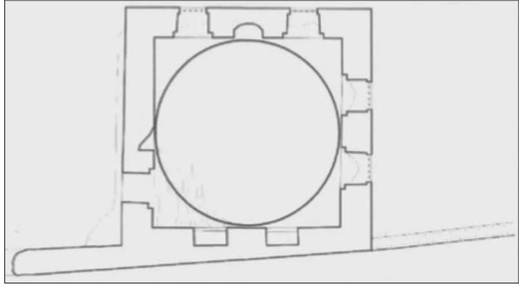
Plan 3. Atik Valide Sultan Sıbyan Mektebi planı (İstanbul Vakıflar II. Bölge Müdürlüğü'nden alınan, 2012 tarihli rölöve analiz raporunda bulunan plan)
