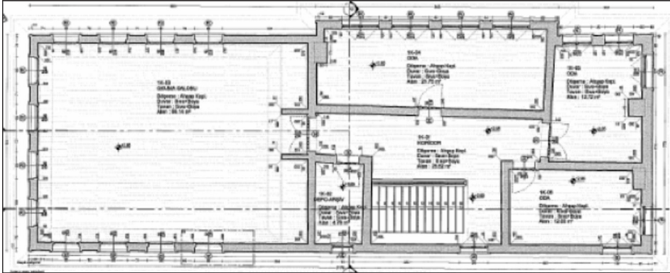
Plan 8. Selimiye Sıbyan Mektebi planı (İstanbul 6 Numaralı Kültür Varlıklarını Koruma Bölge Kurulu Müdürlüğü'nden alınan, 2013 tarihli restorasyon projesinde bulunan plan).
