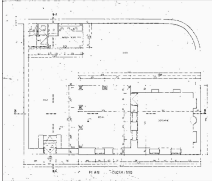
Plan 2. Rüstem Paşa Sıbyan Mektebi Planı (İstanbul 6 Numaralı Kültür Varlıklarını Koruma Bölge Kurulu Müdürlüğü'nden)
