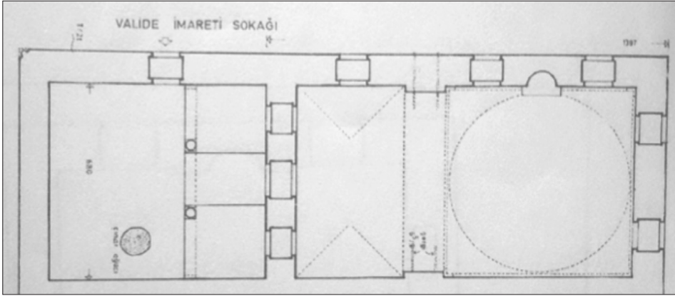
Plan 1. Mihrimah Sultan Sıbyan Mektebi Planı (İstanbul Vakıflar II. Bölge Müdürlüğü'nden alınan, Zeynep Ahunbay'a ait plan)
