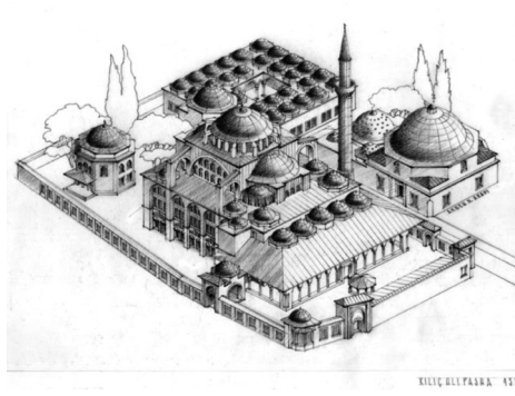
Kılıç Ali Paşa Külliyesi'nin izometrik çizimi.
